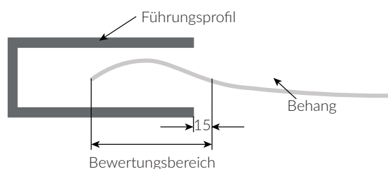
Abb. 55: Bewertungsbereich Behandveränderungen
