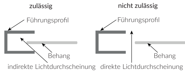
Abb. 52: Lichtdurchscheinungen
