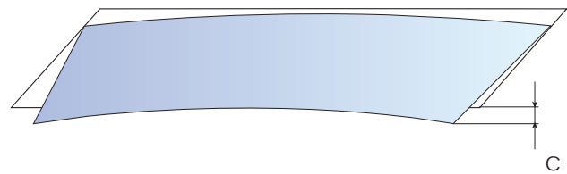
Abb. 45: Säbelförmigkeit
