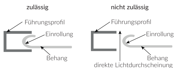
Abb. 54: Zulässige Einrollung
